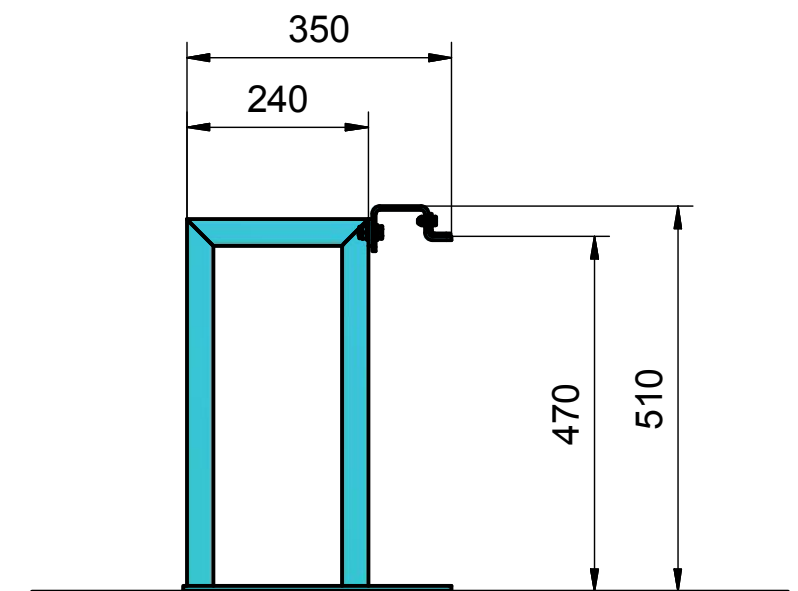
Seitenansicht
